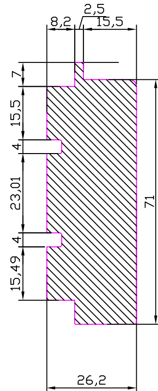
SET DI LEGNI PER FASCIE SPECIALI PER SERIE MODANATA
